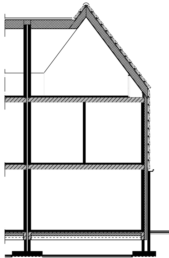
doorsnede 1:100
