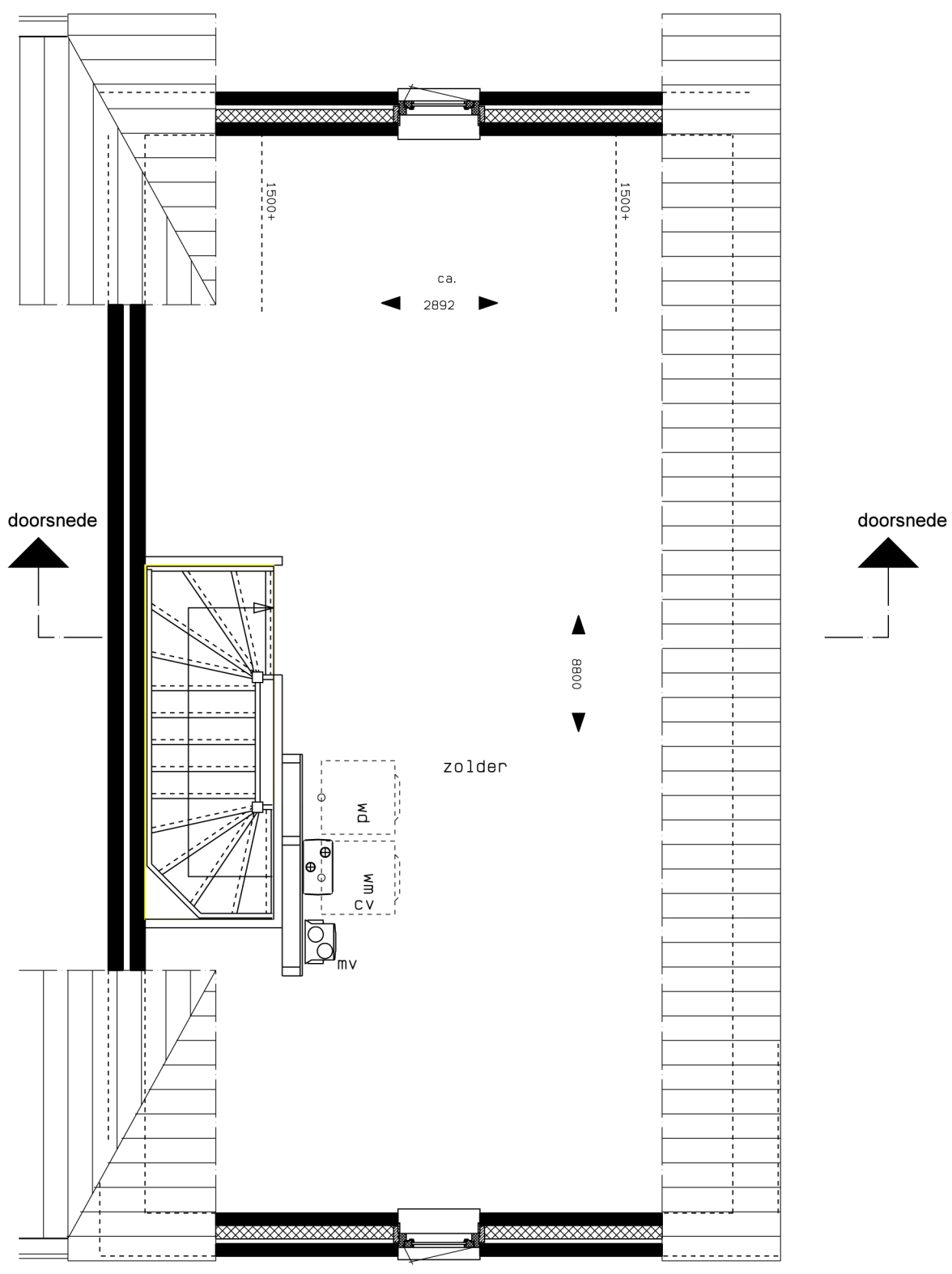
plattegrond zolder 1:50
